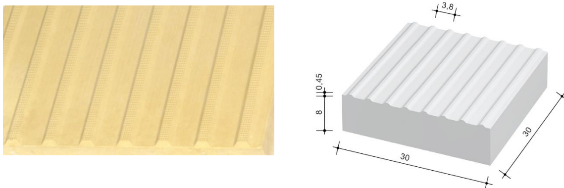
Rys.2. Płytki kierunkowe symetryczne - prowadząca- szczegół powierzchni
