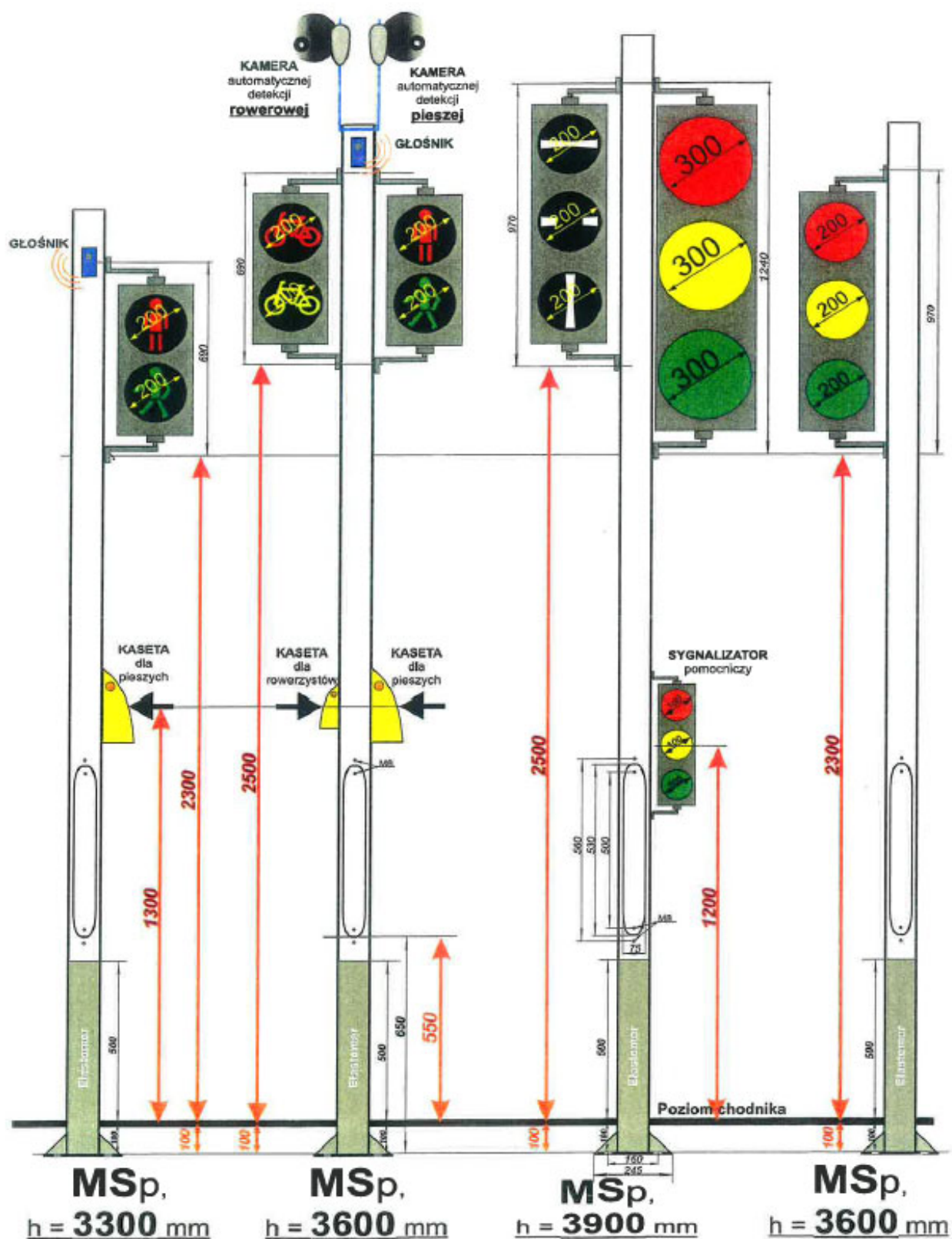
Rys. 2.7. – Sylwetki masztów sygnalizacyjnych
