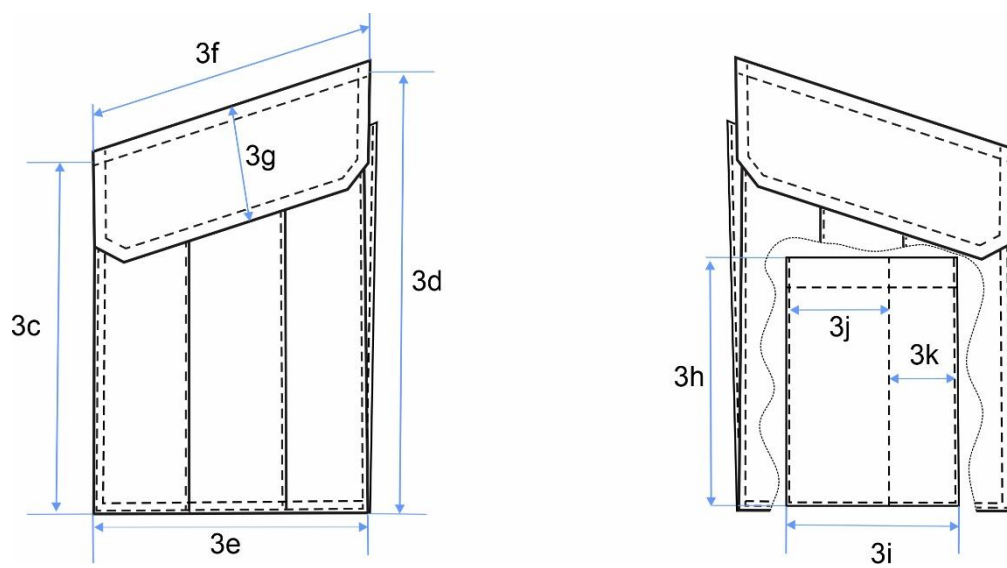
Rysunek 13 Wymiarowanie kieszeni nakładanej i organizera
