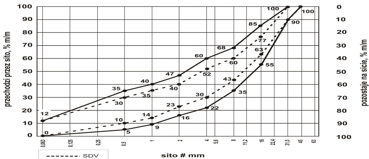
Rysunek 1. Mieszanka niezwiązana 0/31,5 do warstwy z mieszanki niezwiązanej z kruszywem C50/30
